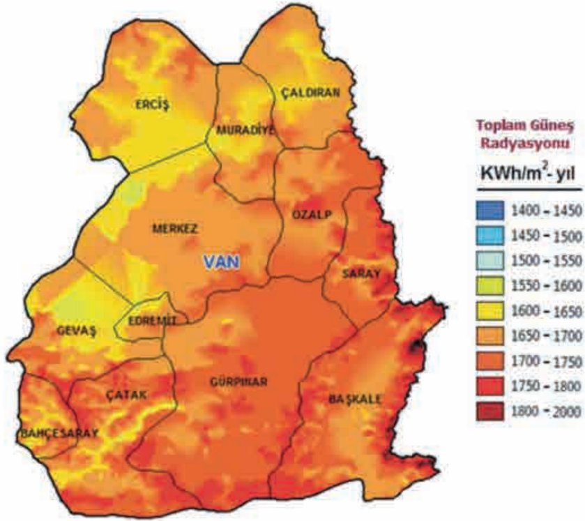
Şekil 10. Van İli Güneş Enerjisi Potansiyel Atlası (GEPA)
