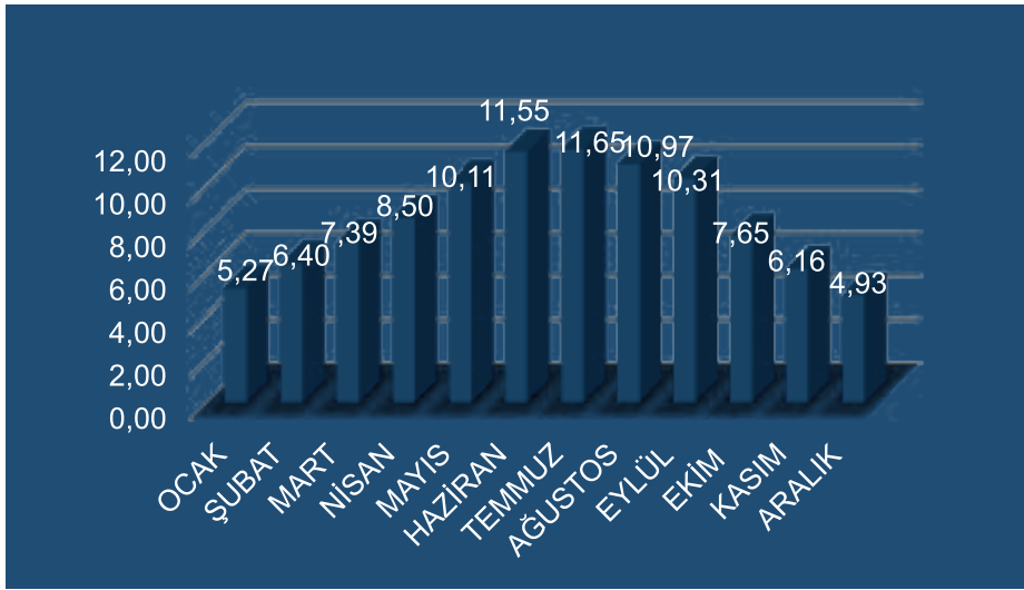
Şekil 12. Van İli’nin aylık bazda ortalama günlük güneşlenme süreleri (GEPA, www.eie.gov.tr )
