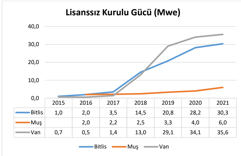
Grafik 77: TRB2 Bölgesi Lisanssız Kurulu Gücü (Mwe)
