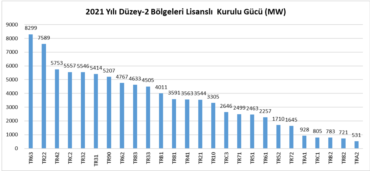
Grafik 73: 2021 Yılı Düzey 2 Bölgeleri Lisanslı Kurulu Gücü (MW)
