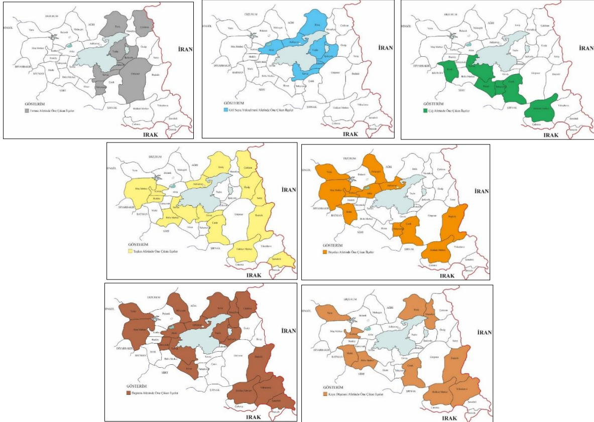
Harita 26: TRB2 Bölgesi İlçelerinde Afet Türlerine Göre Etki Alanı Dağılımları
