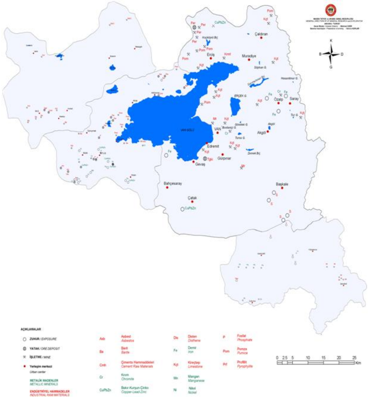
Harita 16: TRB2 Bölgesi Maden Haritası
